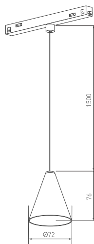
Рис. 1. Чертеж и габаритные размеры
