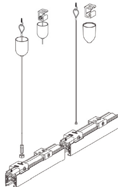
Рисунок 4. Крепление шинопровода с помощью подвесов
